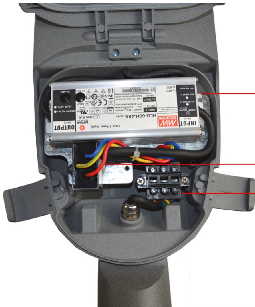
Odgromnik 10kV
